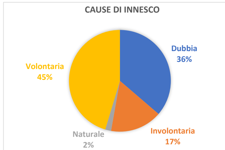
Fig. 1-3 - Ripartizione delle cause di innesco per gli incendi boschivi in Abruzzo nel periodo 2012-2022
