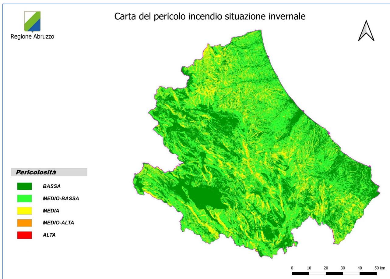
Fig. 4-16 - Carta della pericolosità a valenza nazionale situazione invernale
