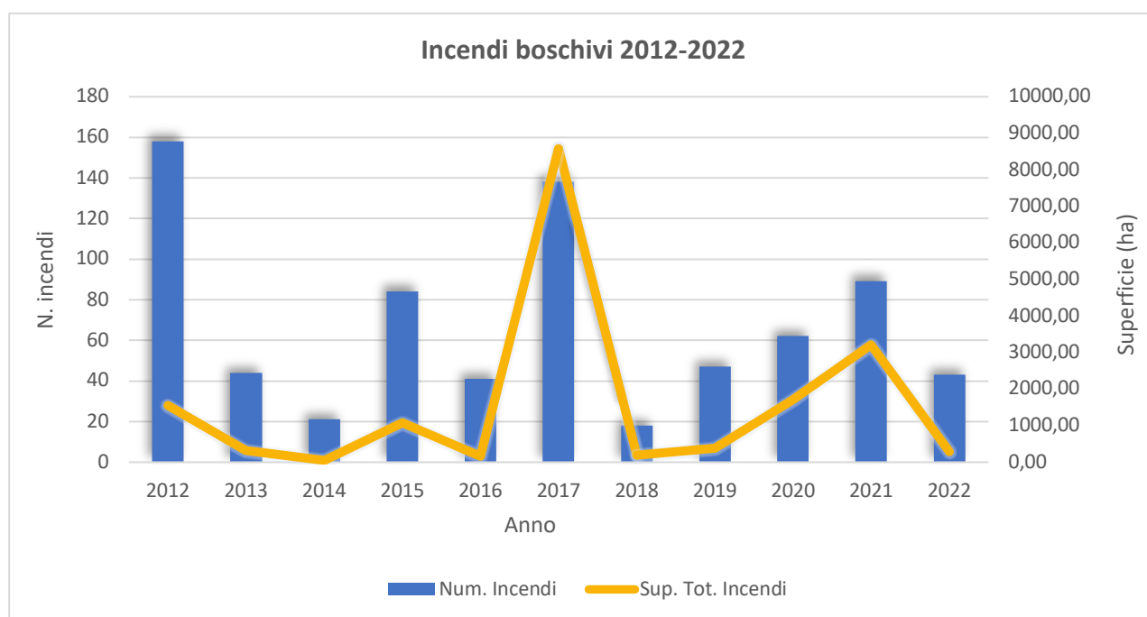
Fig. 1-1 - Andamento annuale del numero di incendi boschivi e delle superfici bruciate (periodo 2012-2022)
