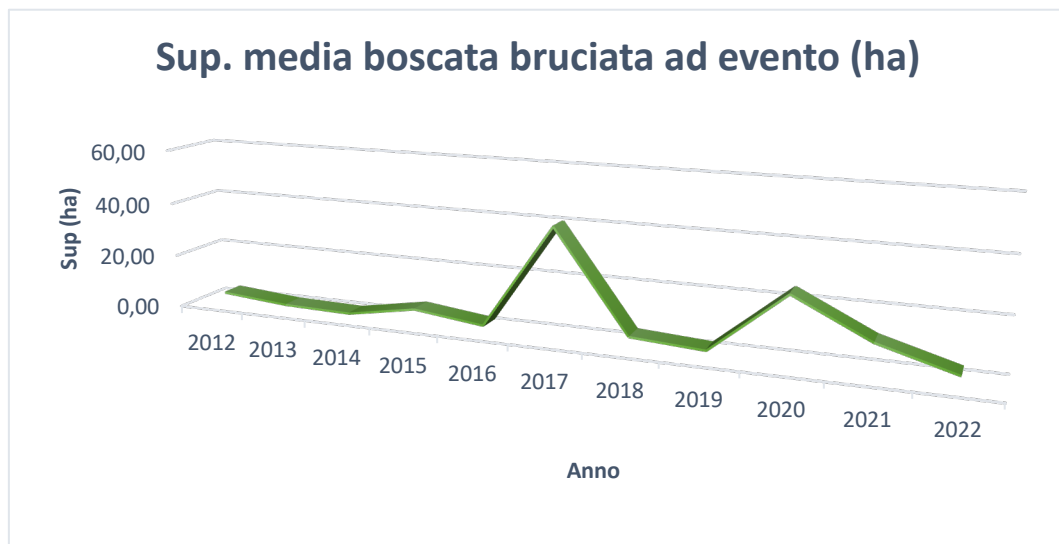
Fig. 1-2 - Andamento annuale superficie boscata media percorsa dal fuoco per evento
