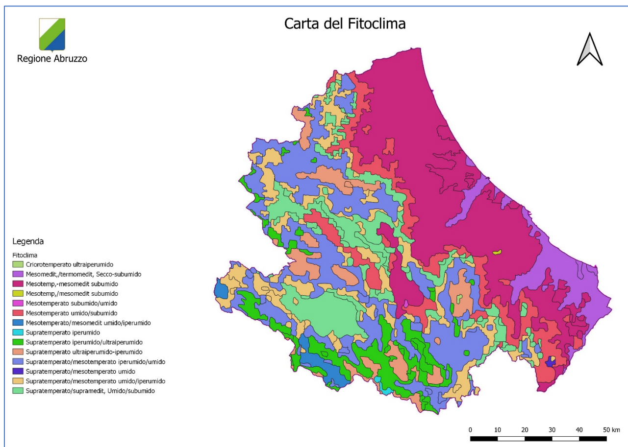
Fig. 4-3 - Carta del fitoclima
