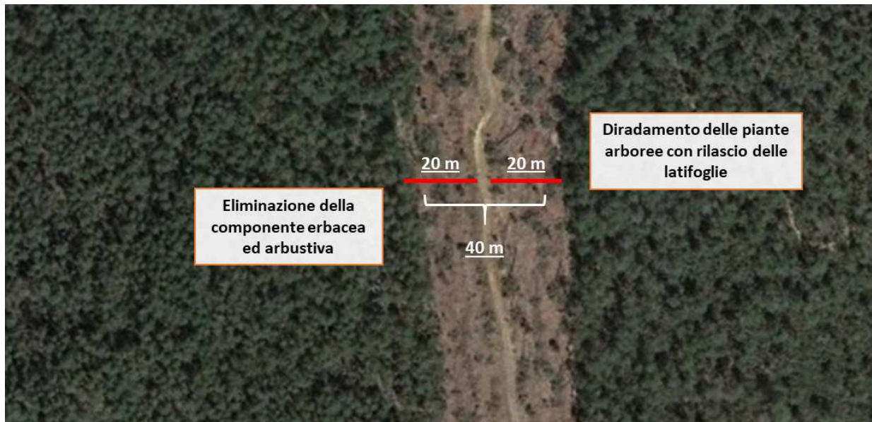
Fig. 5-2 - Viale parafuoco: esempio di viale parafuoco con fasce parafuoco di 20 m per lato
