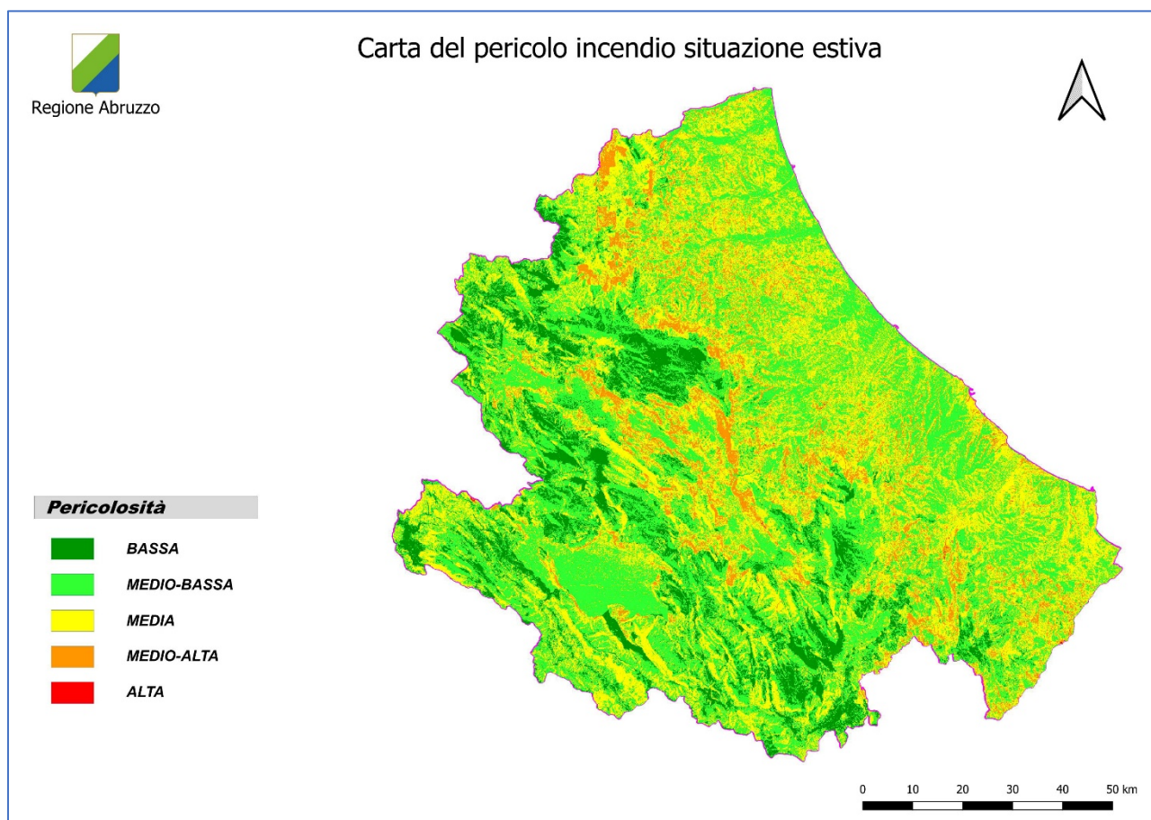
Fig. 4-15 - Carta della pericolosità a valenza nazionale situazione estiva
