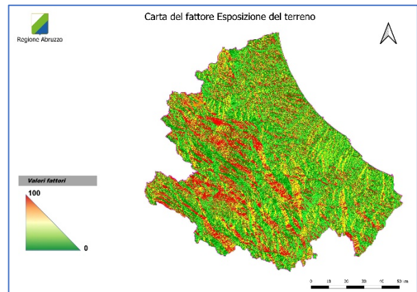
Fig. 4-10 - Carta delle esposizioni del terreno
