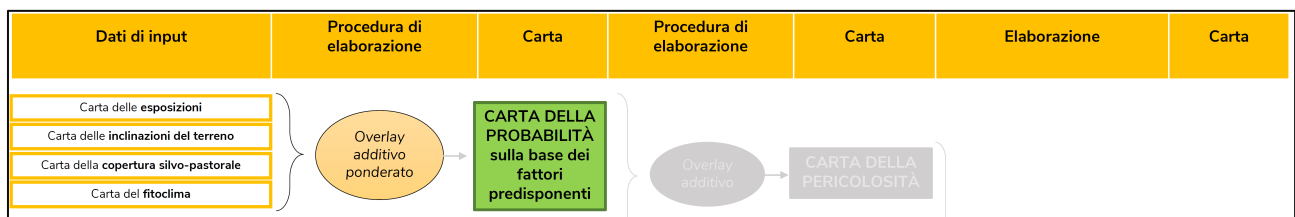
Fig. 4-2 - Schema metodologia elaborazione "Carta della Pericolosità"
