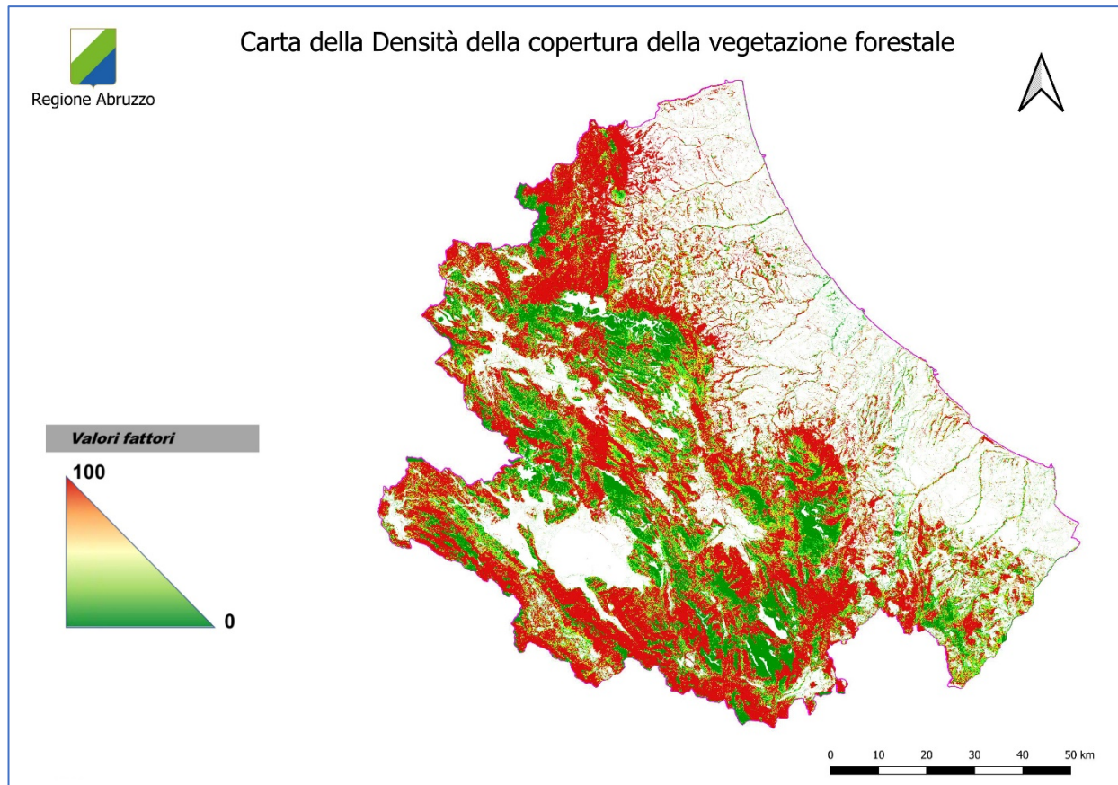
Fig. 4-7 - Carta della percentuale di copertura forestale
