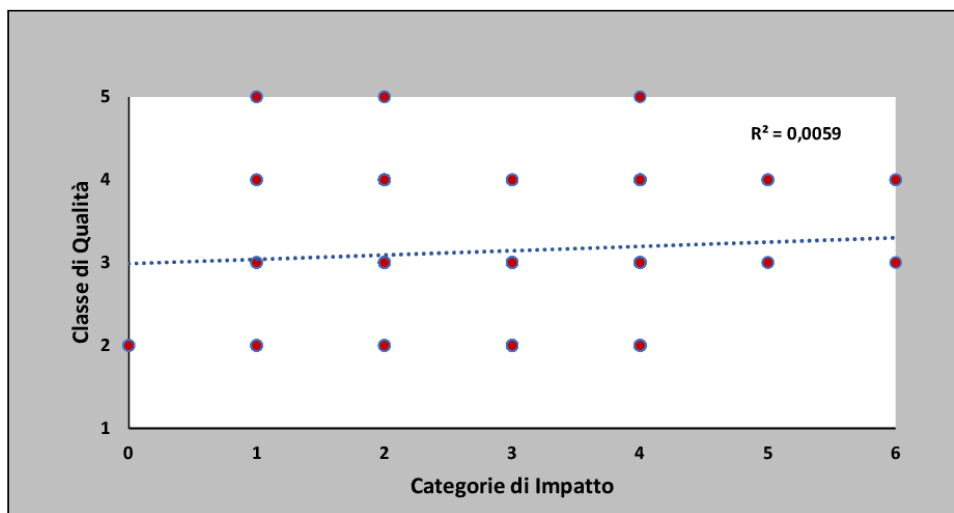
Fig. 6bis - Correlazione tra categorie di impatto e stato di qualità dei CI abruzzesi.
