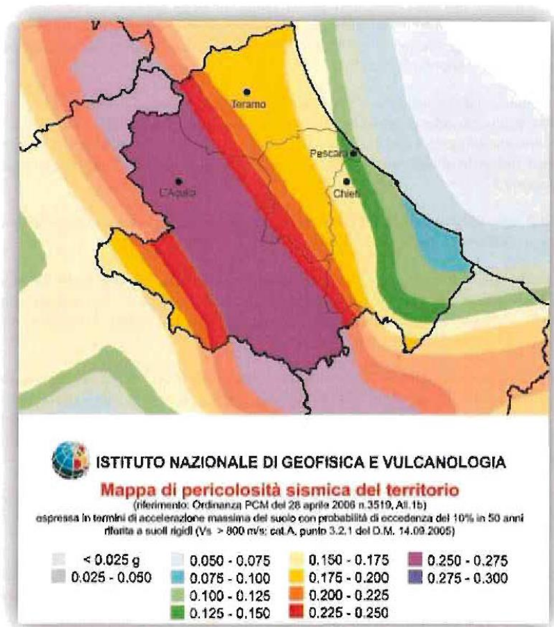
Mappa della pericolosità sismica del territorio - Abruzzo
