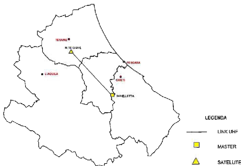
Layout rete radiomobili regionale 118 Abruzzo
