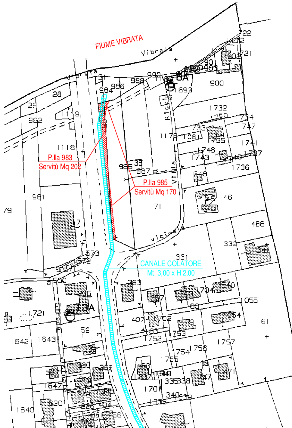
PLANIMETRIA CATASTALE scala 1:2000
