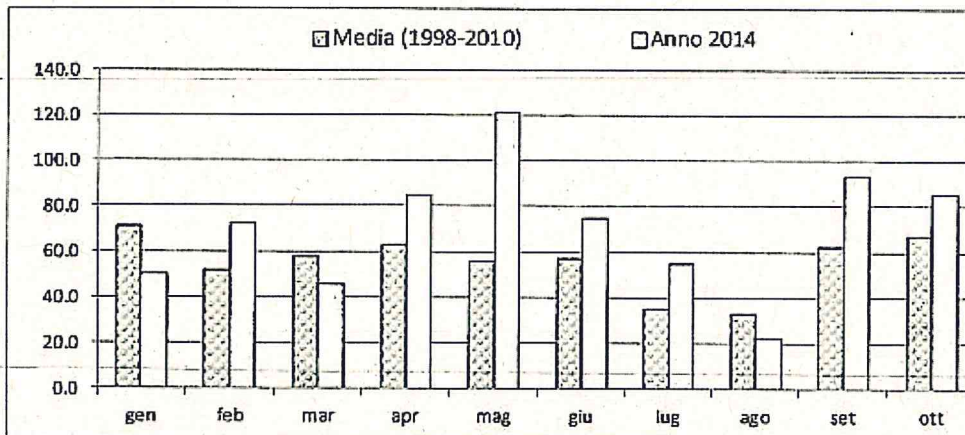
Dati pluviometrici
