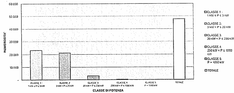
Fig. 3.6 – Numero di impianti in esercizio in Italia per classi di potenza (Fonte GSE)
