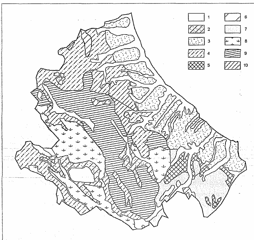
Figura 2.3 - Carta geolitologica
