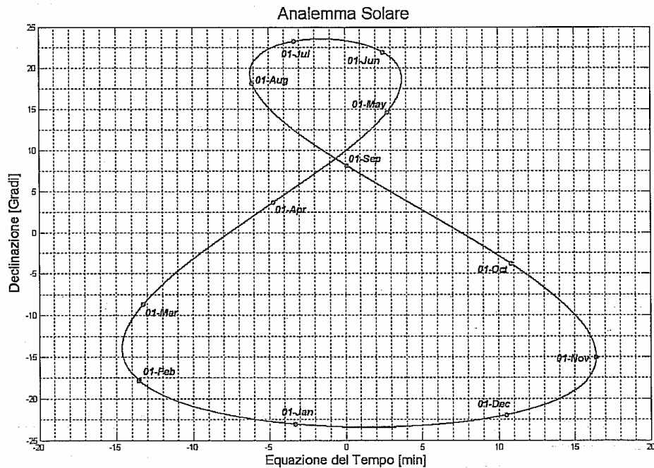
Figura 1.8: Analemma Solare
