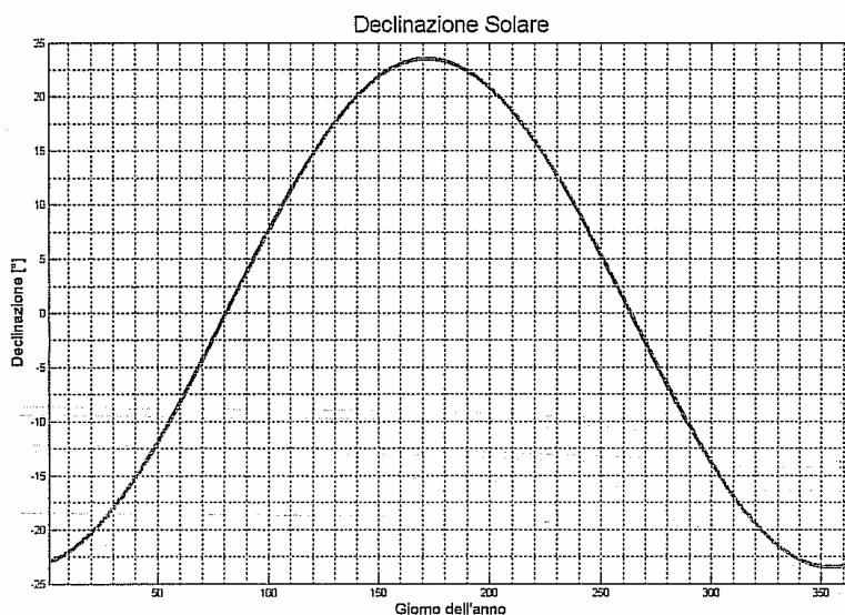
Figura 1.7: Declinazione Solare
